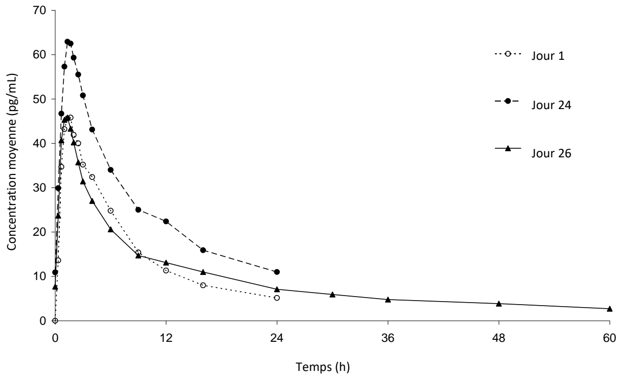
Figure 1 – Courbe de la concentration plasmatique moyenne d'éthinylœstradiol en fonction du temps après l'administration orale de 1 dose unique et de doses multiples de LOLO chez des femmes volontaires en bonne santé (n = 15)
