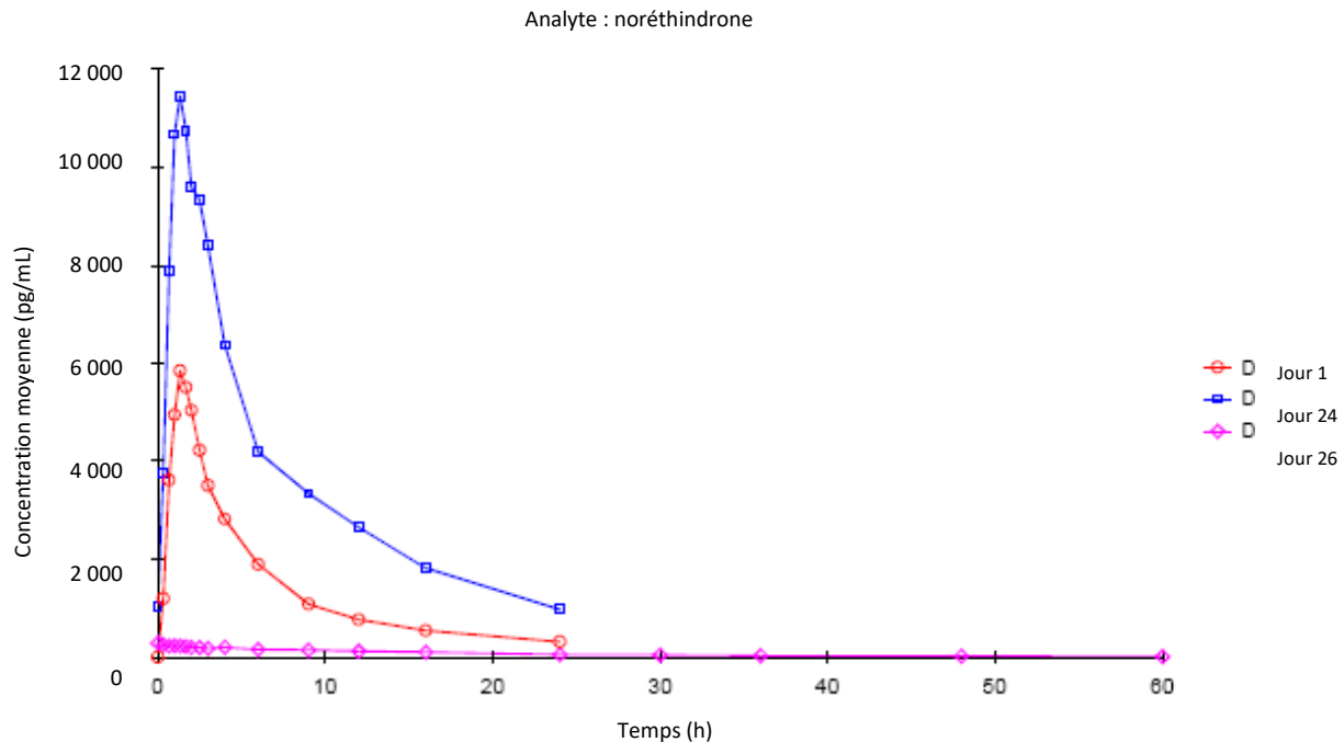
Figure 2 – Courbe de la concentration plasmatique moyenne de noréthindrone en fonction du temps après l'administration orale de 1 dose unique et de doses multiples de LOLO chez des femmes volontaires en bonne santé (n = 15)
